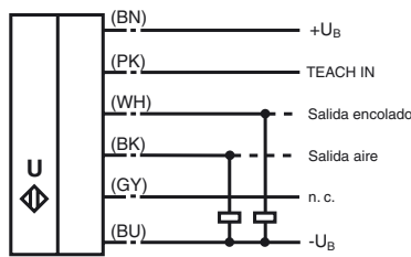
Símbolo normalizado/conexión: Control de hoja doble
